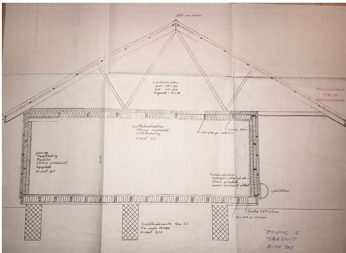
Tværsnit Spinning fra 2011.
